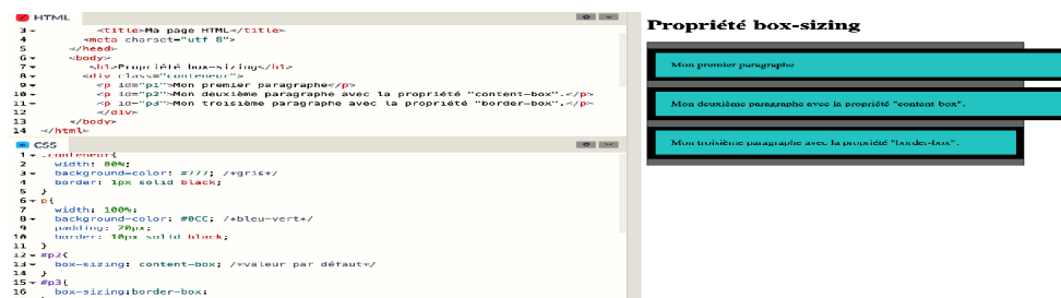
FIGURE 3.19 – Exemple d’utilisation de la propriété box-sizing
