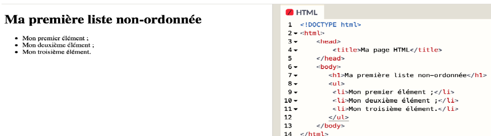
FIGURE 2.8 – Exemple de liste non-ordonnée
