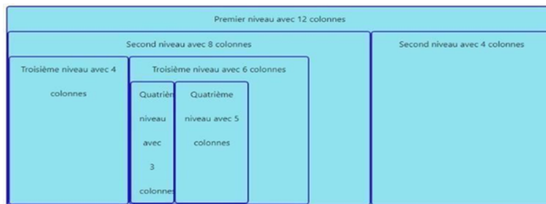
FIGURE 11.3 – Exemple de mise en page 2 sous Bootstrap4
