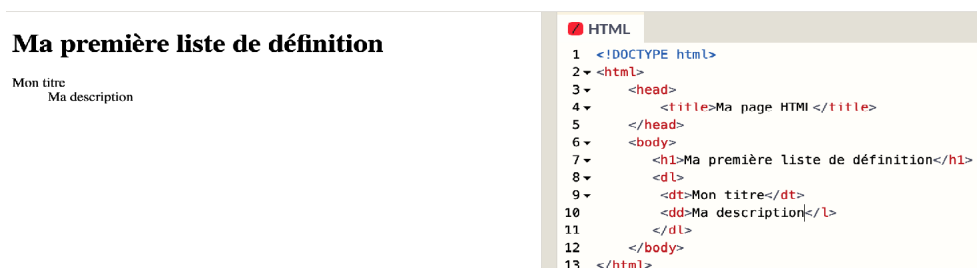
FIGURE 2.10 – Exemple de liste de définition
